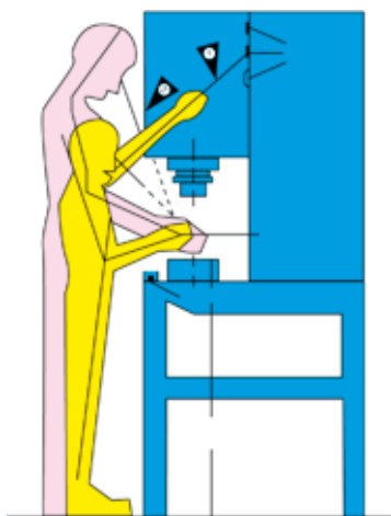
Abb. 2 Maßliche Gestaltung von Steharbeitsplätzen entsprechend den Körpermaßen der Nutzer
