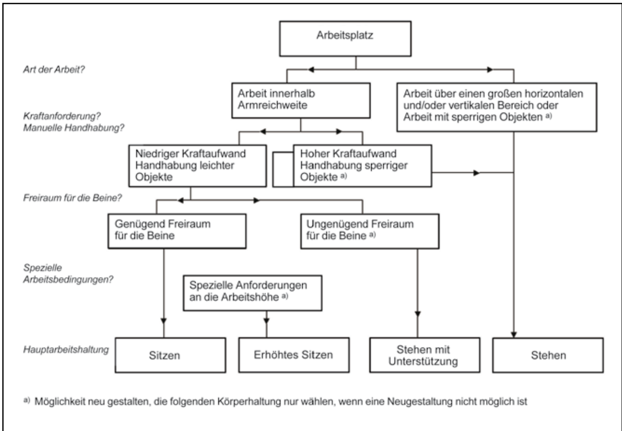
Abb.1 Bestimmung der Hauptarbeitshaltung /23/
